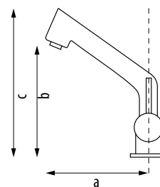
Rozměry a/b/c
